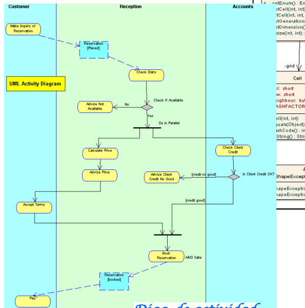
Diag. de actividad
